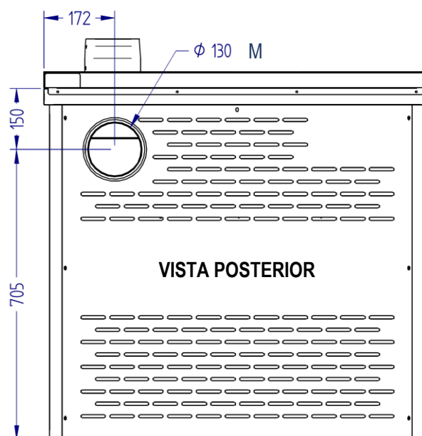
MODELO CON SALIDA DE HUMOS POSTERIOR
