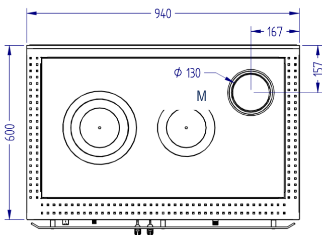
MODÈLE AVEC SORTIE DE FUMÉES SUPÉRIEURE
