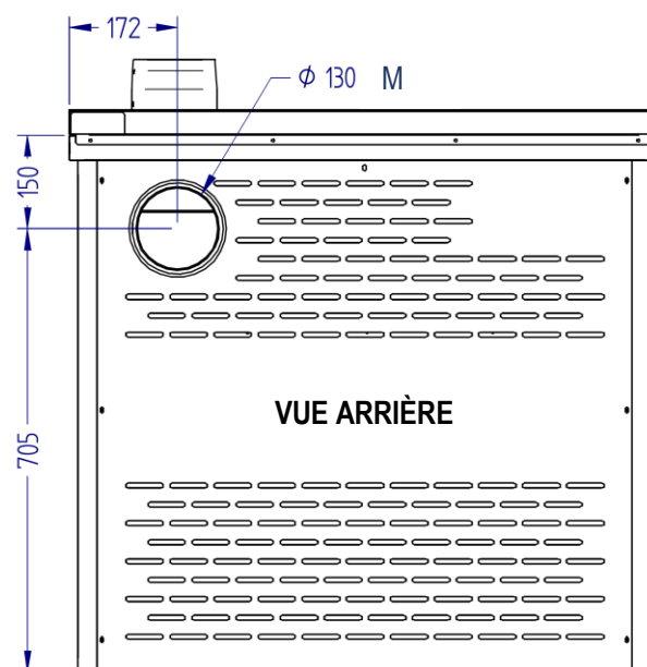
MODÈLE AVEC SORTIE DE FUMÉES POSTÉRIEURE
