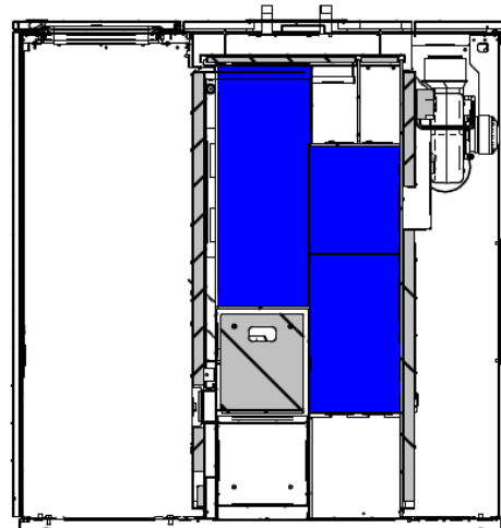
SEZIONE FRONTALE
