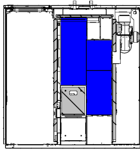
SEZIONE FRONTALE
